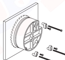
Montage encastré
