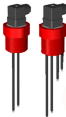
Détecteur avec électrodes coupables à longueur souhaitée
