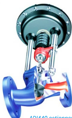
ARI440 actionneur pneumatique
