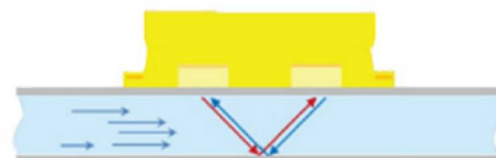
Principe de mesure par ultrasons
