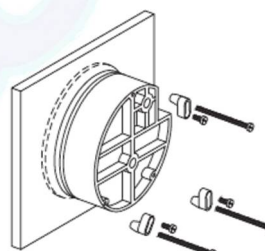
Montage encastré
