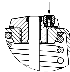
Échappement spécial Numéro K 6996
