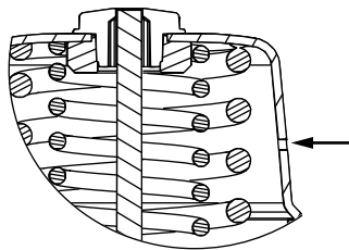
Standard-Entlüftungsbohrung
