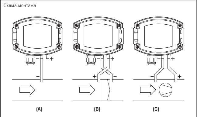
Схема монтажа
