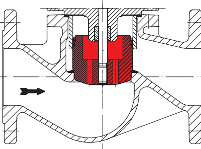
Clapet parabolique avec système d'équilibrage
