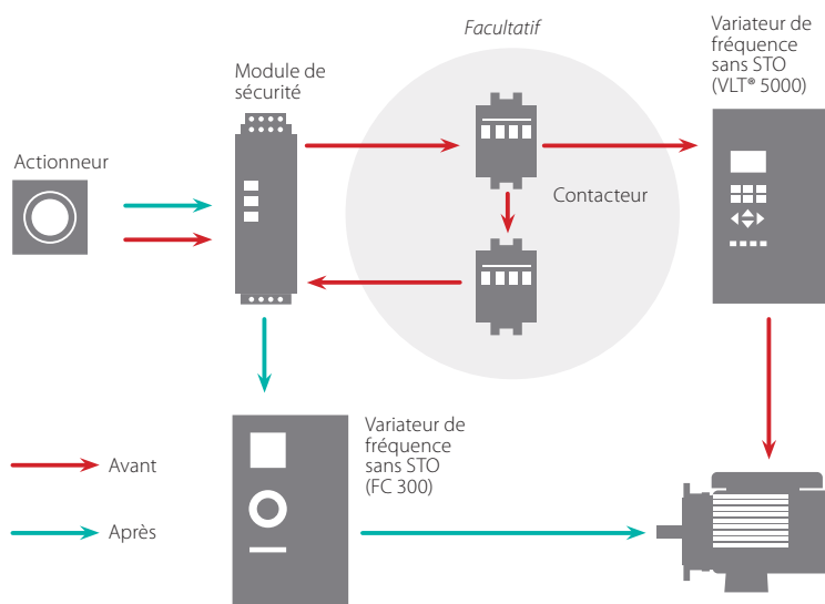
Il est possible de se passer des deux contacteurs sur les installations grâce la fonction de sécurité installée sur le VLT® AutomationDrive.
