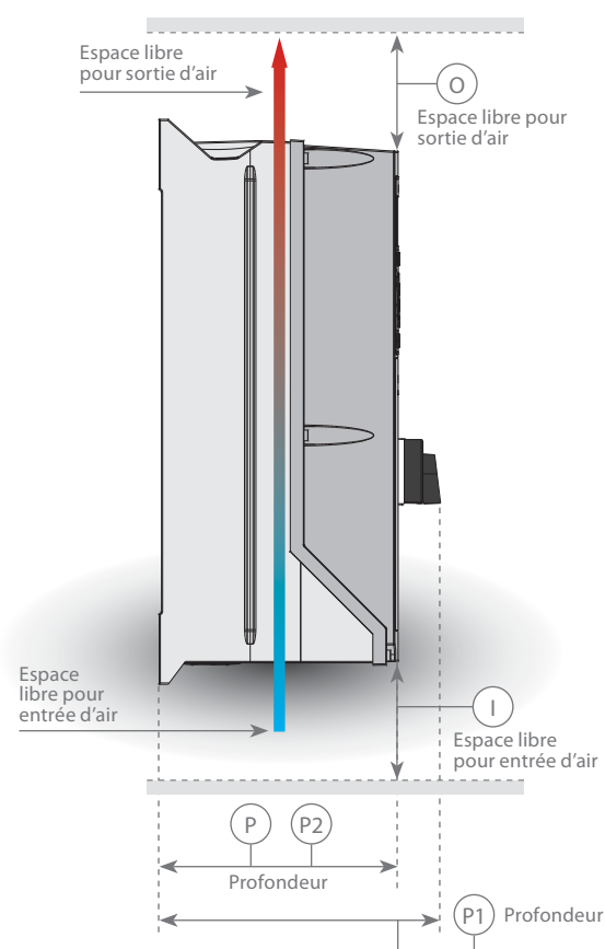
A4 IP 55 avec interrupteur d'alimentation
