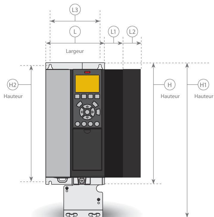
A3 IP 20 avec option C
